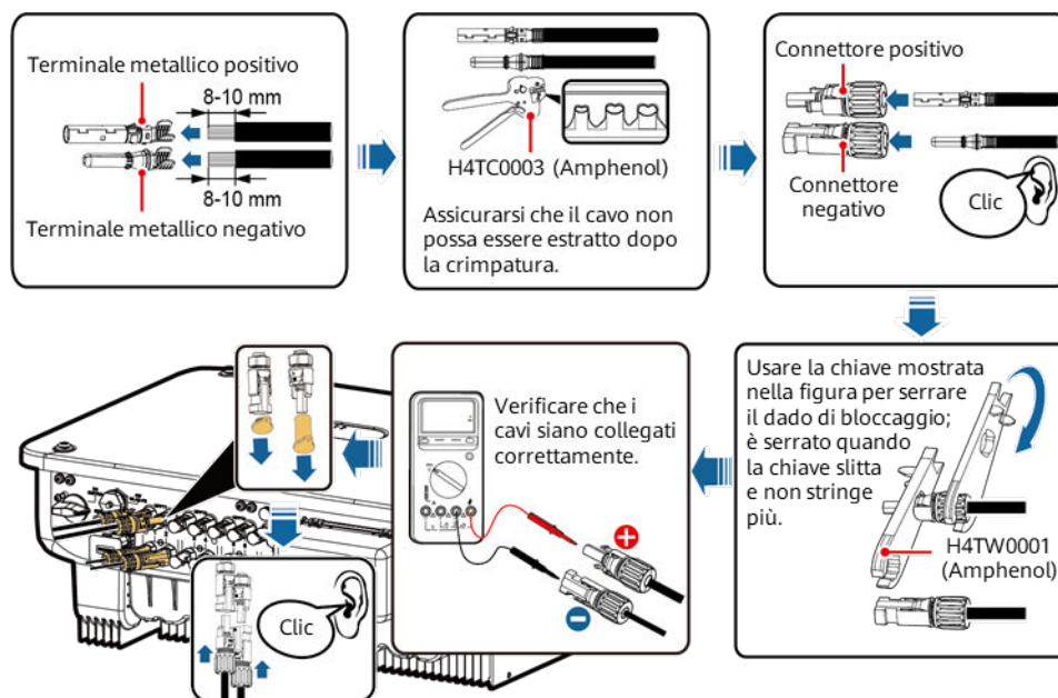
Figura 5-12 Collegamento del cavo di alimentazione CC
