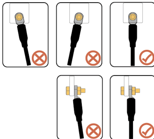
Figura 5-10 Requisiti di cablaggio
