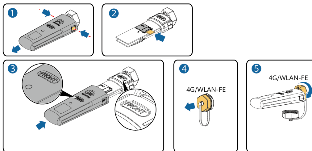
Figura 5-14 Installazione di uno Smart Dongle 4G (SDongleA-03)
