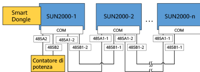
Figura 5-20 Collegamento in rete dello Smart Dongle
