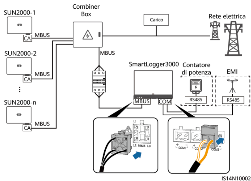
Figura 5-23 Comunicazione MBUS (scenari commerciali e industriali in Cina)
