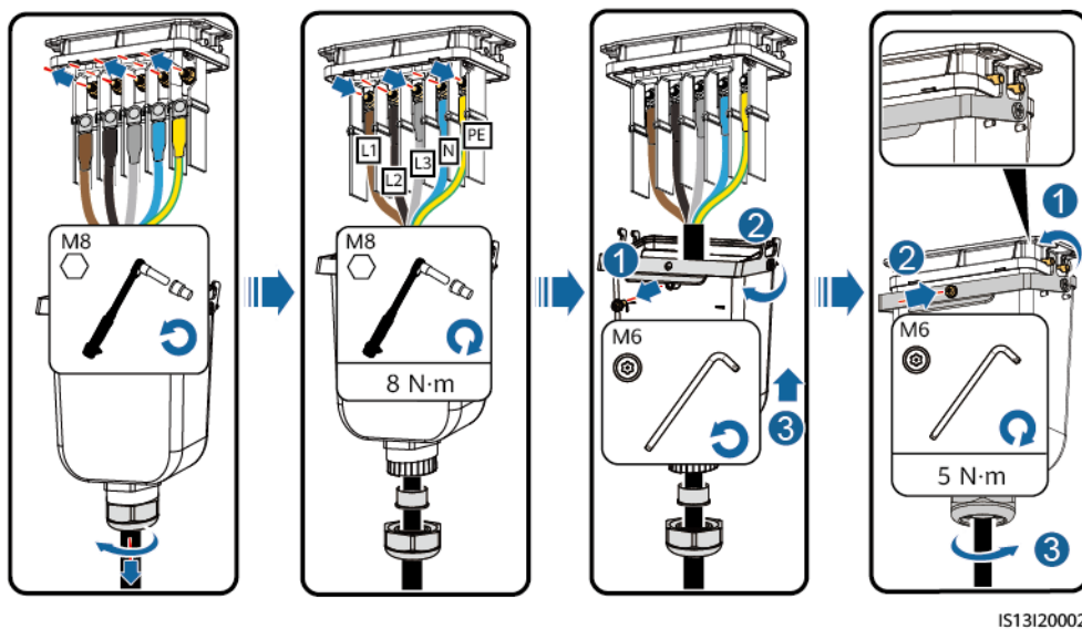
Figura 5-6 Cavo a cinque anime (L1, L2, L3, N e PE)
