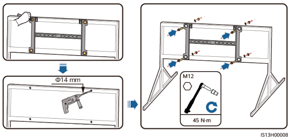
Figura 4-11 Fissaggio della staffa di montaggio
