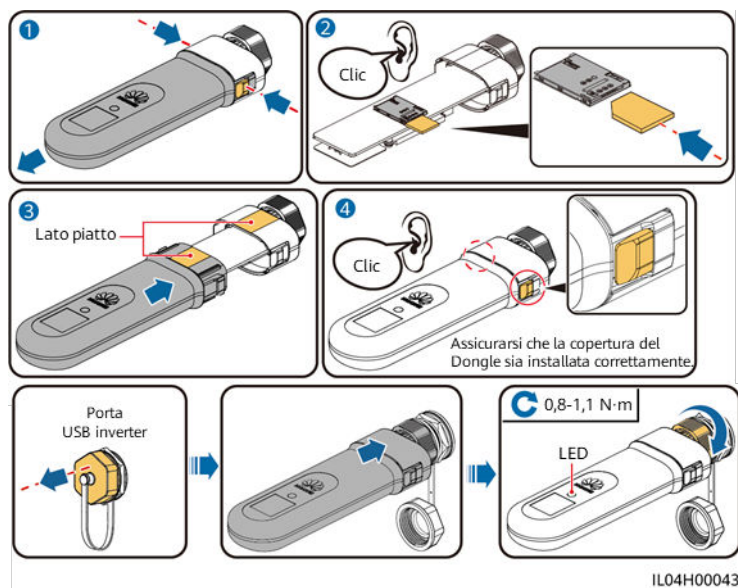
Figura 5-15 Installazione di uno Smart Dongle 4G (SDongleB-06)
