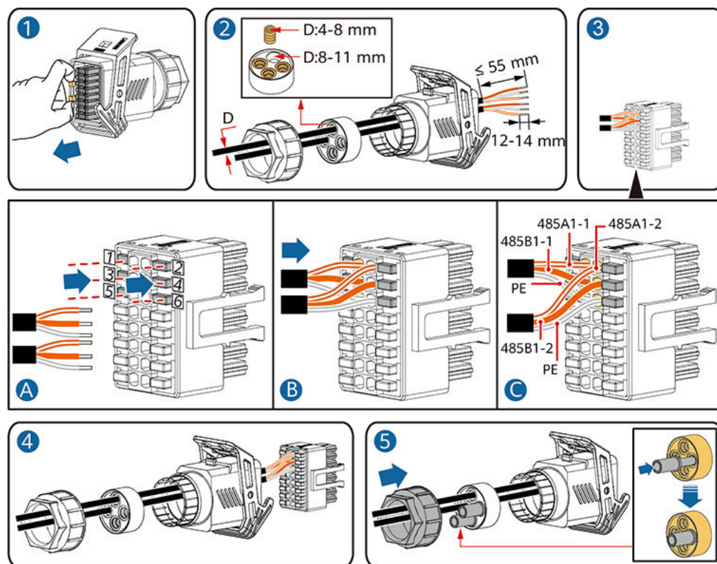
Figura 5-24 Collegamento del cavo
