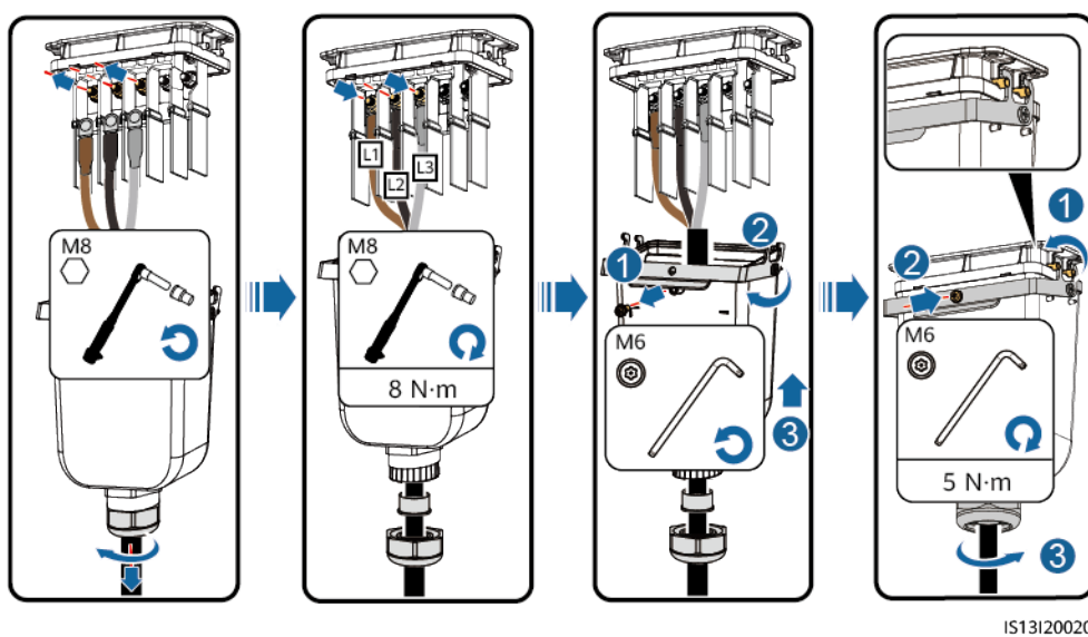
Figura 5-9 Cavo a tre anime (L1, L2 e L3)
