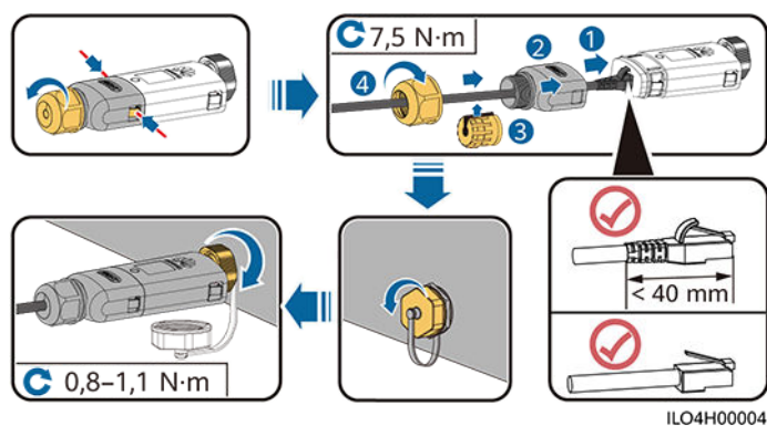
Figura 5-17 Installazione di uno Smart Dongle WLAN-FE (per comunicazioni FE)
