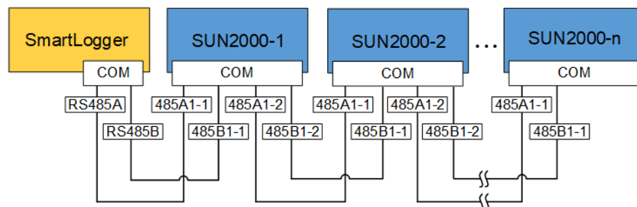
Figura 5-21 Rete SmartLogger
