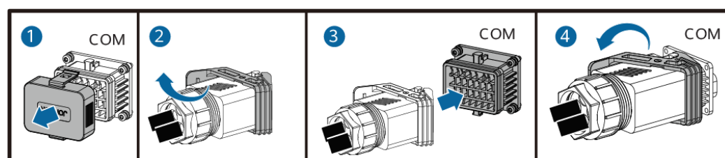
Figura 5-25 Fissaggio del connettore del cavo di segnale
