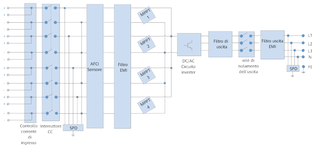
Figura 2-5 Diagramma dello schema
