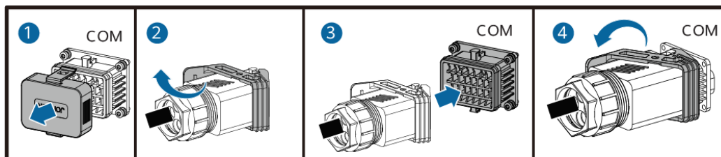
Figura 5-29 Fissaggio del connettore del cavo di segnale
