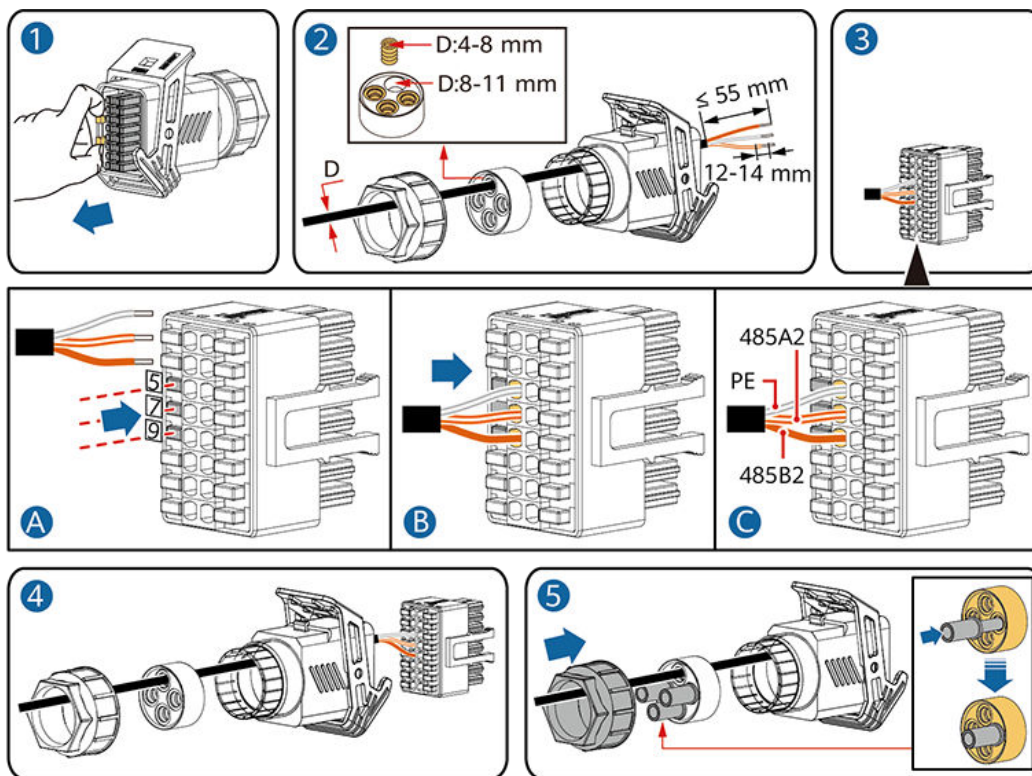
Figura 5-26 Collegamento del cavo
