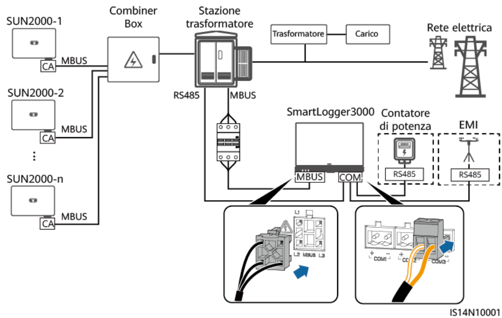
Figura 5-22 Comunicazione MBUS (scenari su scala industriale)
