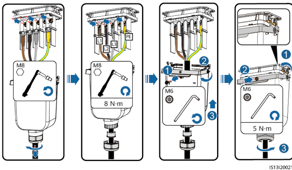
Figura 5-7 Cavo a quattro anime (L1, L2, L3 e PE)
