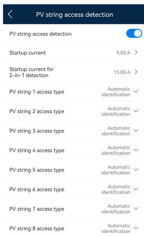
Figura H-1 Rilevamento accesso stringa
