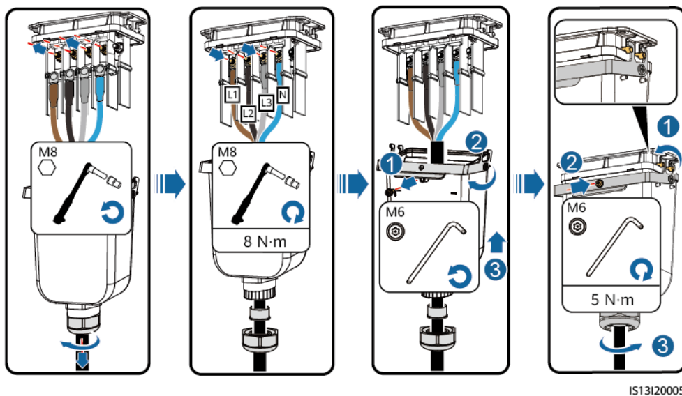
Figura 5-8 Cavo a quattro anime (L1, L2, L3 e N)
