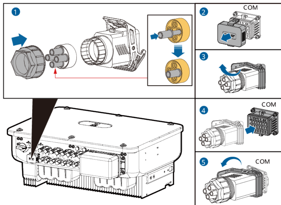
Figura 5-19 Fissaggio del connettore del cavo di segnale
