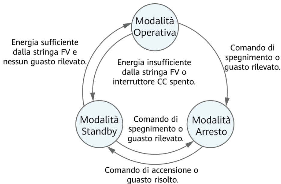
Figura 2-6 Modalità di funzionamento
