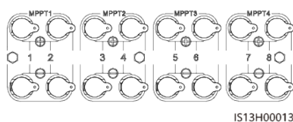
Figura 5-11 Terminali in entrata CC
