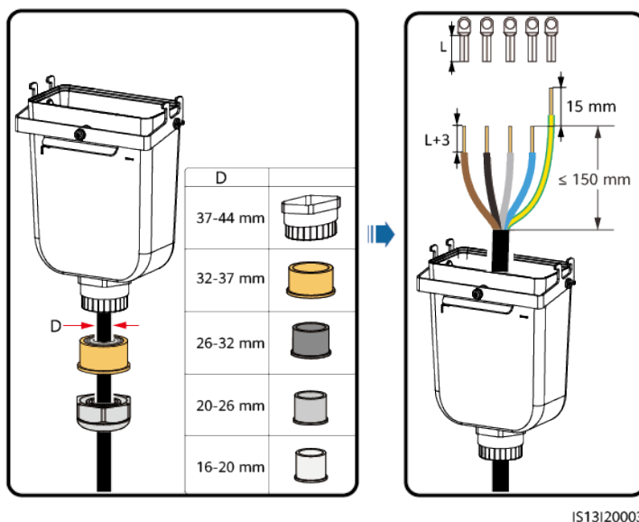
Figura 5-5 Spelatura del cavo di alimentazione CA (viene utilizzato un cavo a cinque anime come esempio)
