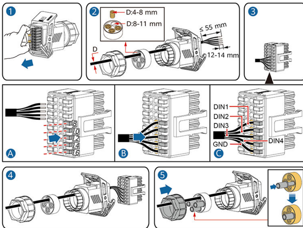
Figura 5-28 Collegamento del cavo
