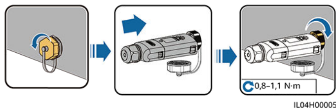
Figura 5-16 Installazione di uno Smart Dongle WLAN-FE (per comunicazioni WLAN)
