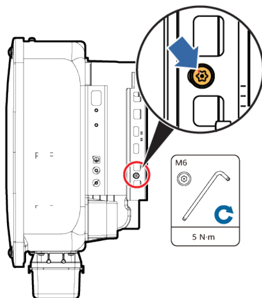
Figura 4-16 Serrare il dado
