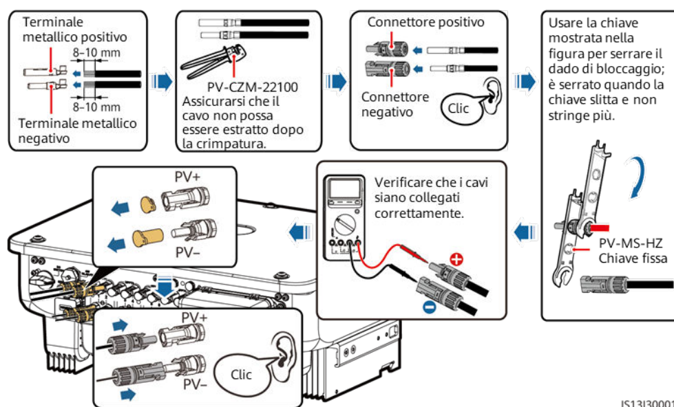
Figura 5-13 Collegamento del cavo di alimentazione CC
