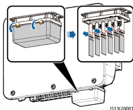
Figura 5-4 Rimozione della morsettiera CA
