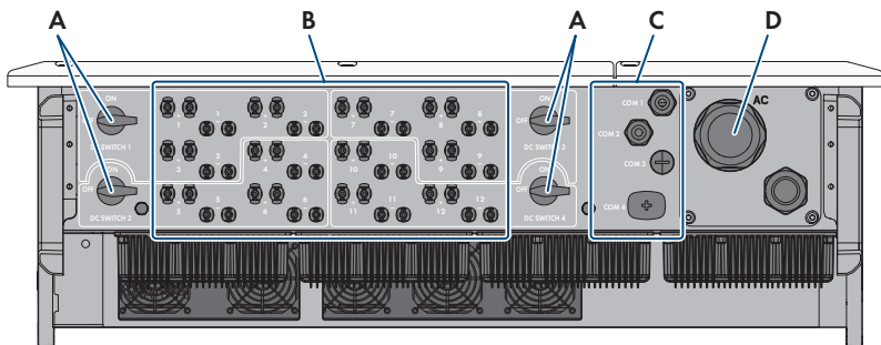
Abbildung 7: Gehäuseöffnungen an der Unterseite des Wechselrichters
