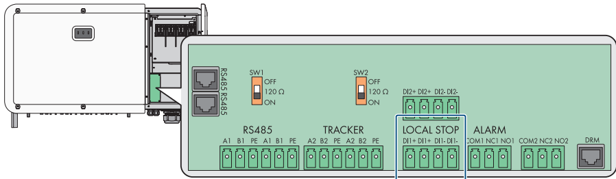
Abbildung 10: Digitale Eingänge für die Schnell-Stopp-Funktion auf der COM-Baugruppe
