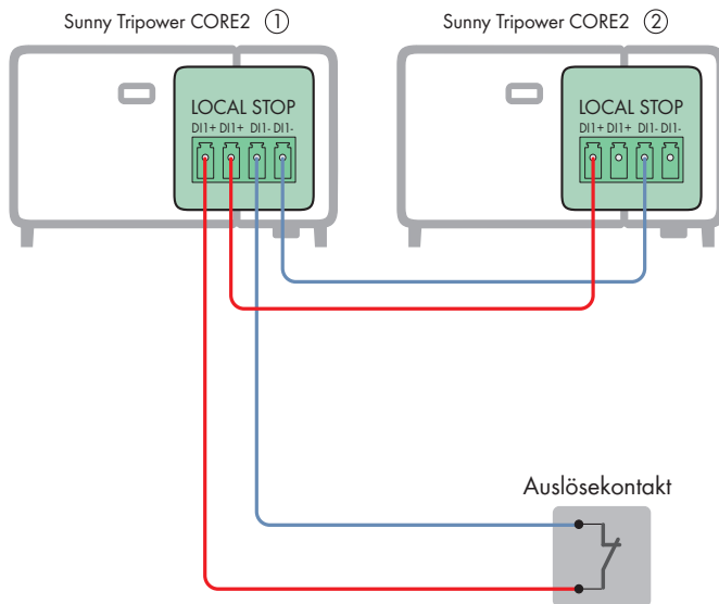
Abbildung 11: Verschaltungsübersicht für den Anschluss eines Kontakts für den Schnell-Stopp und der Verbindung mehrerer Wechselrichter
