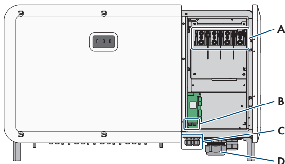
Abbildung 8: Anschlussbereiche im Inneren des Wechselrichters
