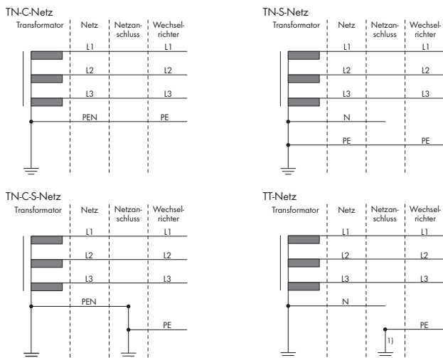
Abbildung 6: Übersicht der zugelassenen Netzformen
