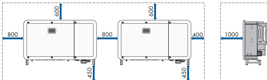
Abbildung 4: Empfohlene Abstände (Maßangaben in mm)
