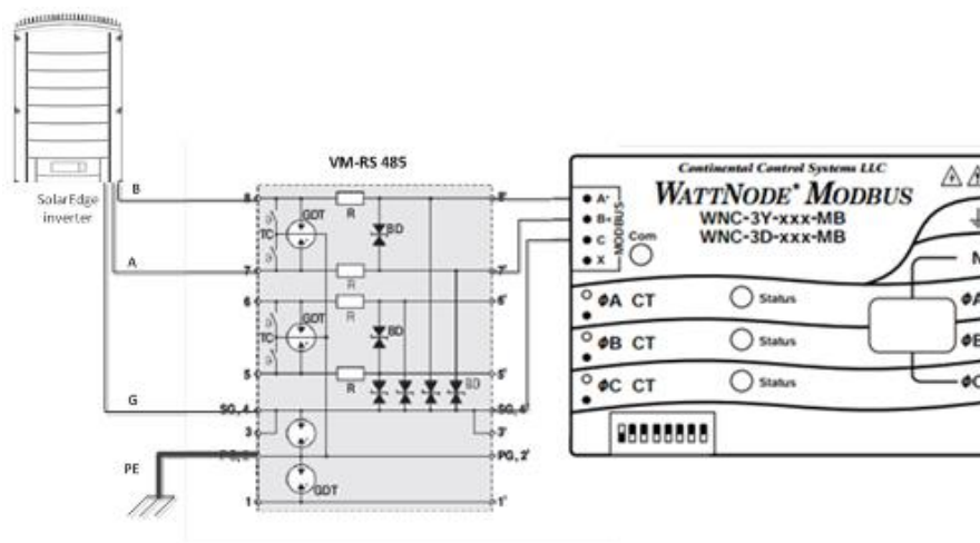
Abbildung 12: Anschluss von Schutzvorrichtungen
