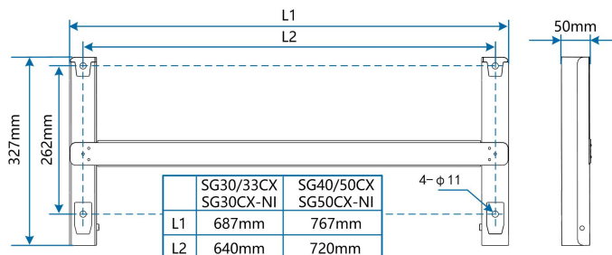
Figure 4-1 Dimensions du support de montage
