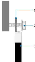
Figure 5-2 Branchement du câble en aluminium
