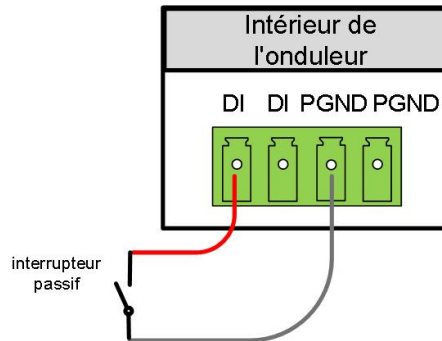
Figure 5-9 Contact d'arrêt local
