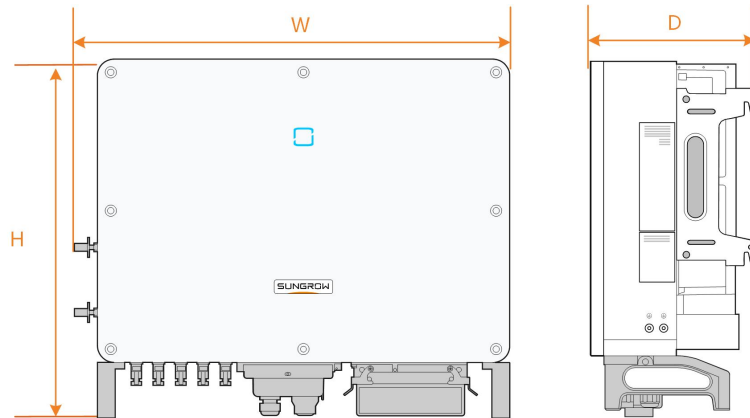
Figure 2-3 Dimensions de l'onduleur (en mm)
