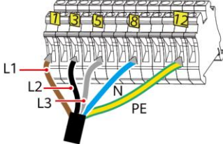
Borne côté Backup Box (triphase)
