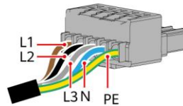
Borne côté onduleur (triphase)
