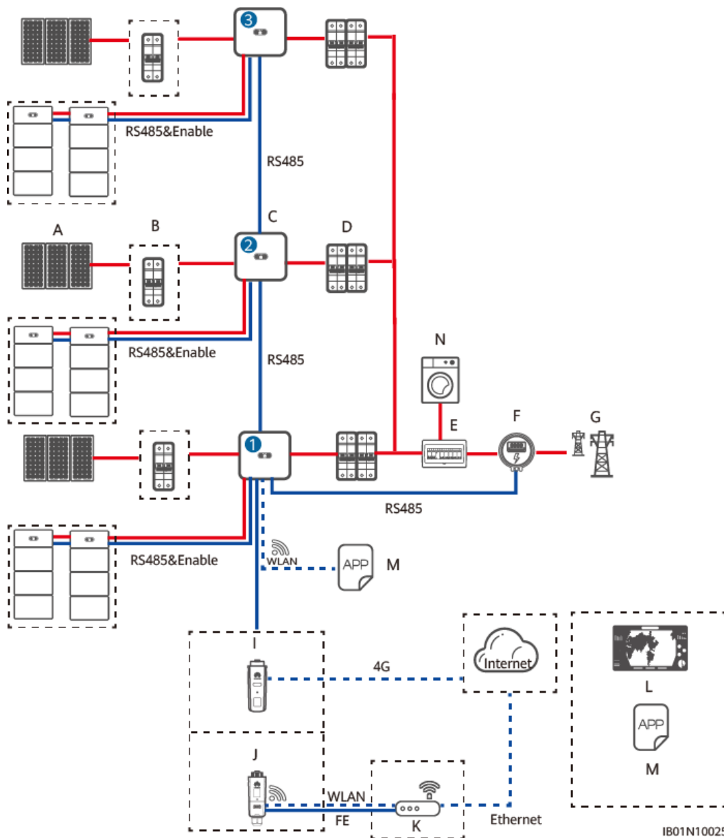
Figure 4-3 Mise en réseau du Smart Dongle (composants optionnels indiqués par des cadres en pointillés)
