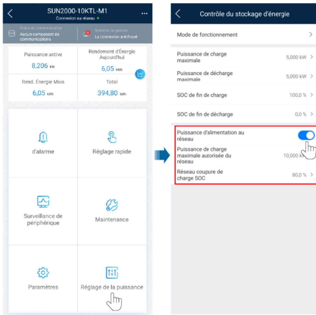
Figure 4-8 Réglage des paramètres de contrôle du stockage d'énergie
