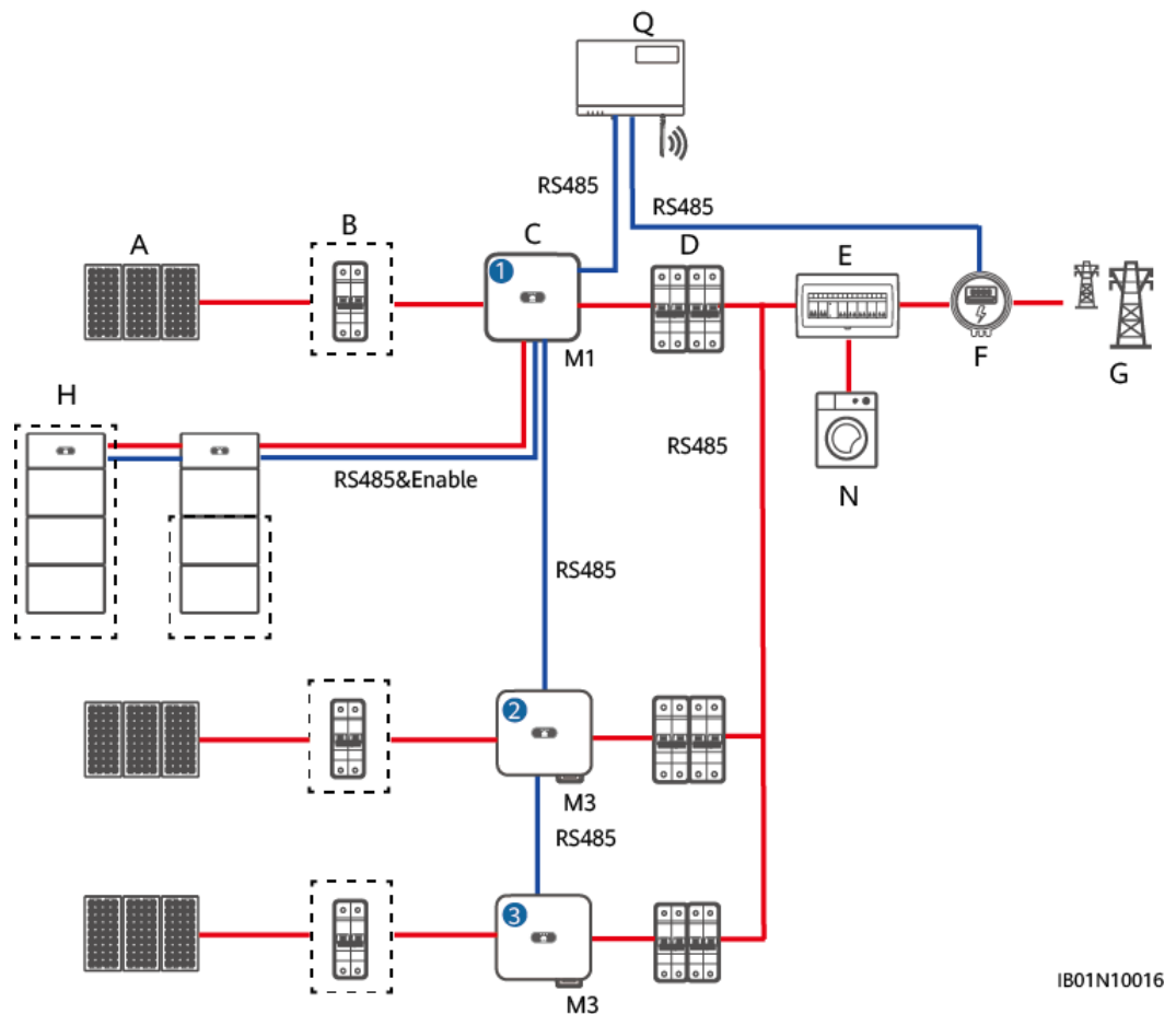
Figure 4-2 Mise en réseau d'un onduleur SUN2000-(3KTL-10KTL)-M1 et de deux onduleurs SUN2000-(20KTL, 29.9KTL, 30KTL, 36KTL, 40KTL)-M3 (composants optionnels indiqués par des cadres en pointillés)
