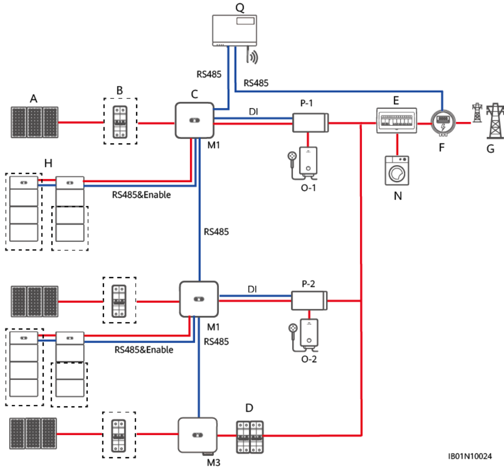
Figure 4-12 Mise en réseau de deux onduleurs SUN2000-(3KTL-10KTL)-M1 et d'un onduleur SUN2000-(20KTL, 29.9KTL, 30KTL, 36KTL, 40KTL)-M3 (composants optionnels indiqués par des cadres en pointillés)
