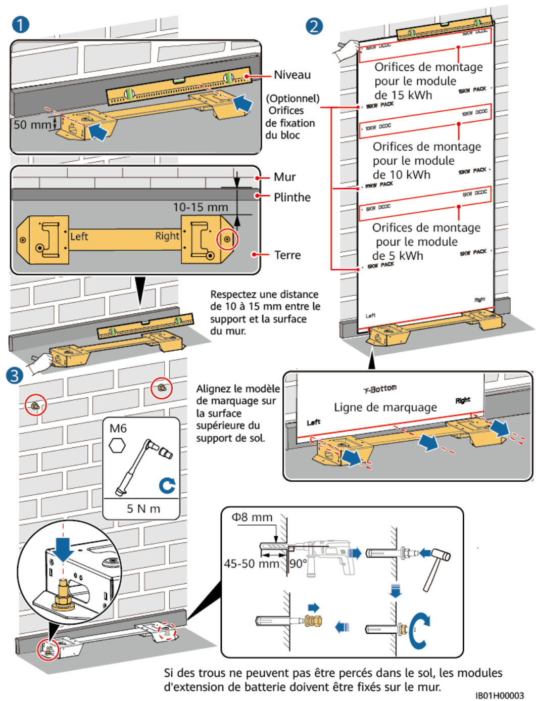
Figure 5-4 Installation des boulons à expansion
