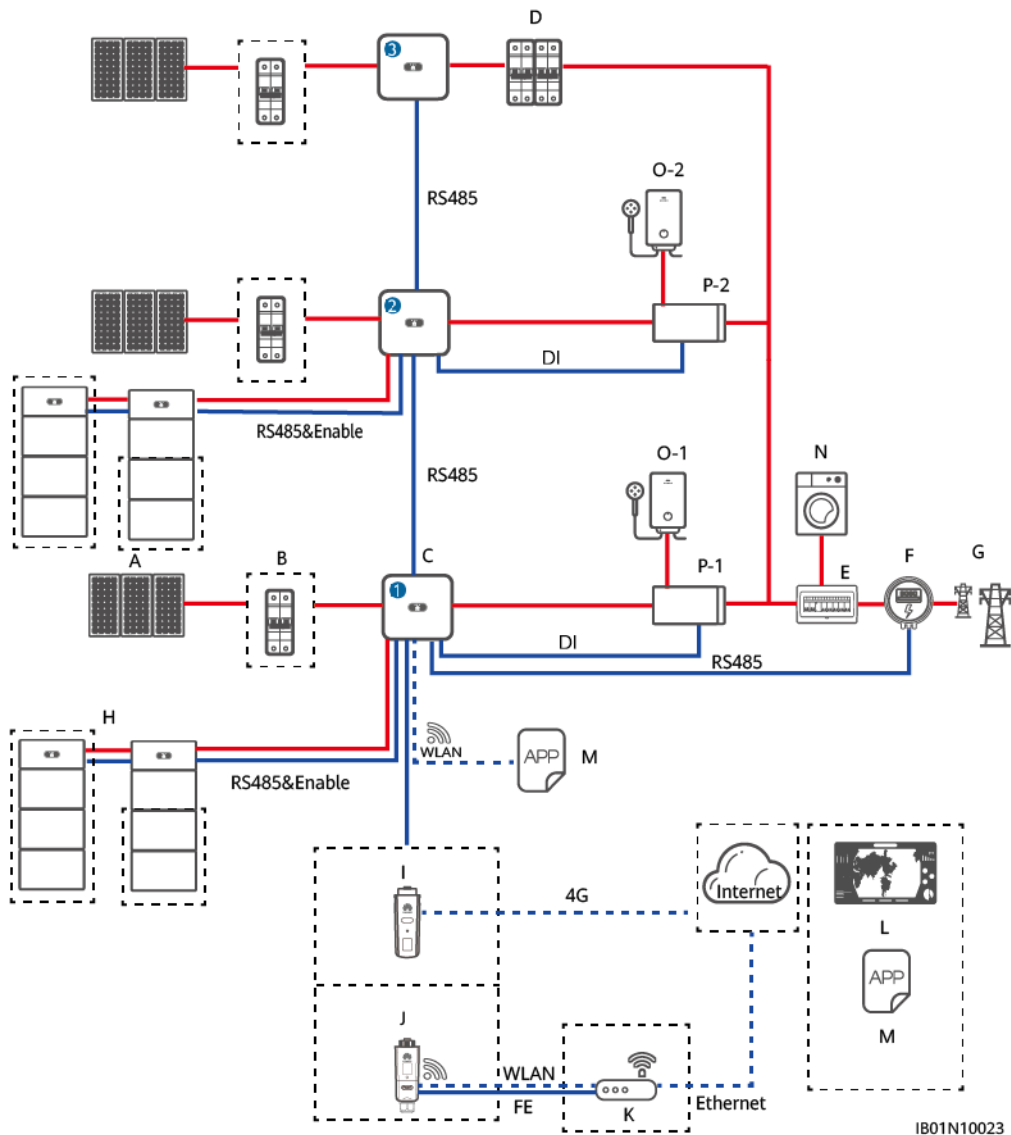
Figure 4-13 Mise en réseau du Smart Dongle dans un ESS raccordé au réseau et hors réseau (composants optionnels indiqués par des cadres en pointillés)
