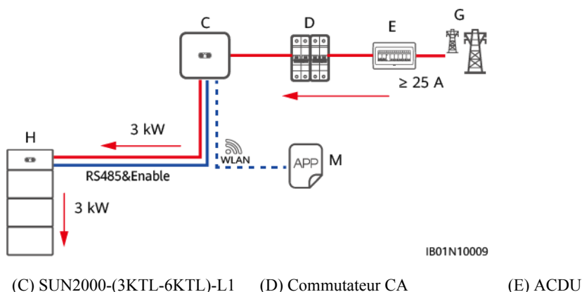
Figure 8-2 Schéma de mise en réseau pour un scénario de source d'alimentation monophasée
