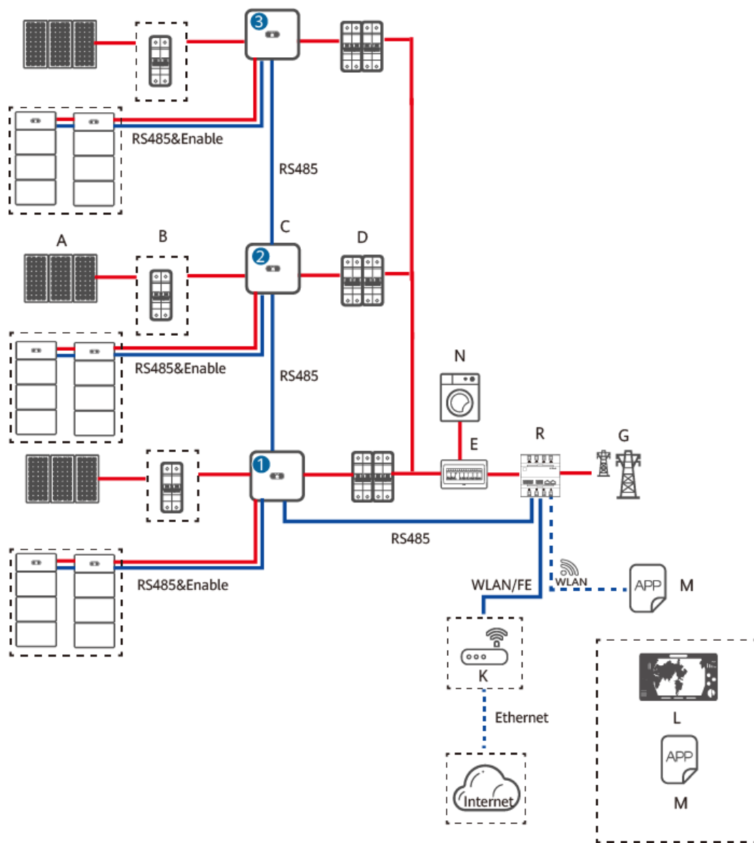
Figure 4-4 Mise en réseau de l'EMMA
