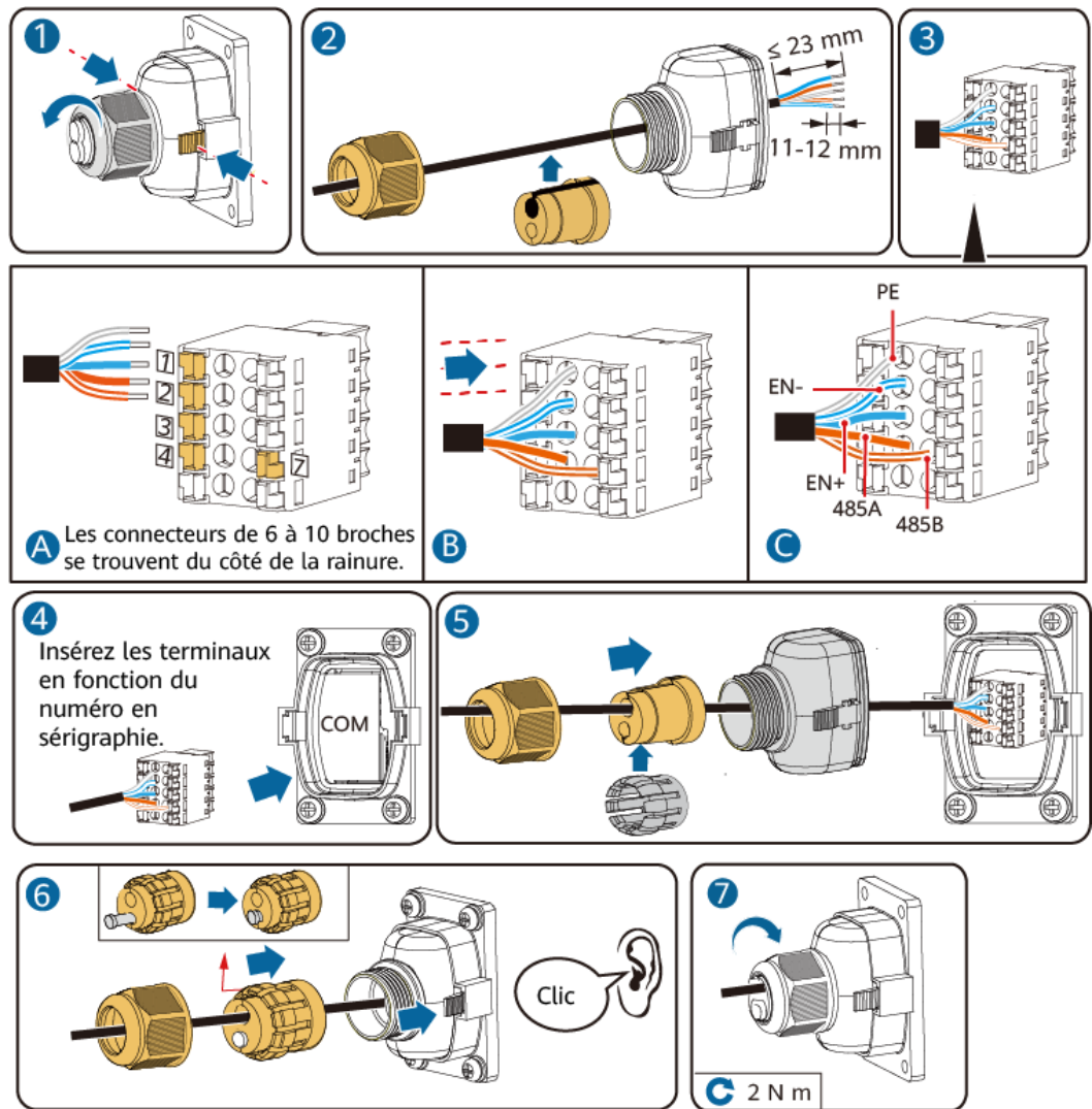
Figure 6-15 Raccordement des bornes de l'onduleur
