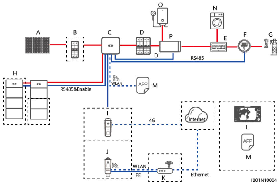
Figure 4-11 Mise en réseau de base de l'ESS hors réseau parallèle (composants optionnels indiqués par des encadrés en pointillé)
