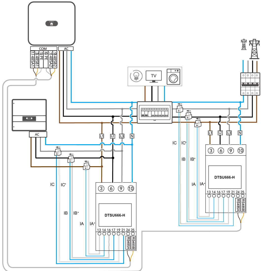
Figure 4-19 Raccordement des câbles du compteur électrique pour le SUN2000-(3KTL-10KTL)-M1
