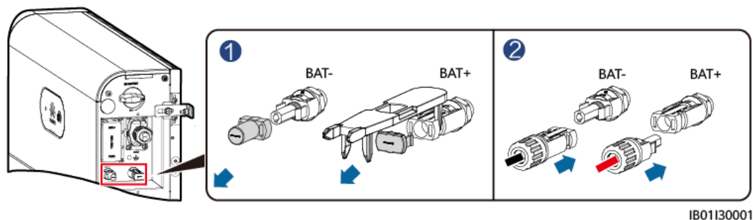
Figure 6-12 Raccordement des câbles de batterie
