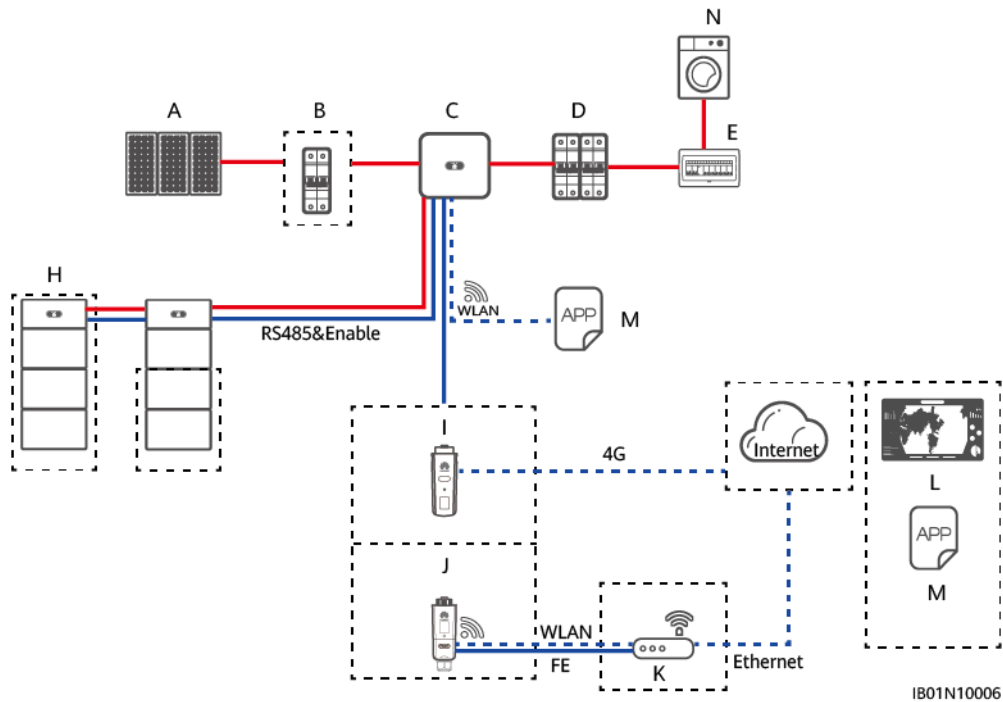
Figure 4-15 ESS hors réseau (composants optionnels indiqués par des encadrés discontinus)
