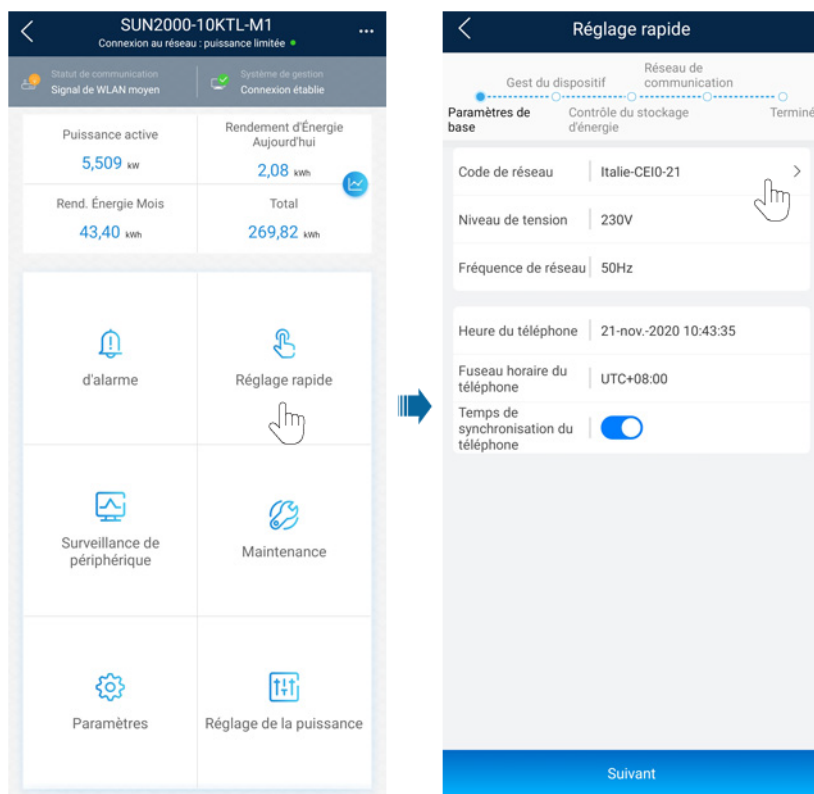
Figure 4-16 Réglage du code de réseau électrique hors réseau (Island-Grid)
