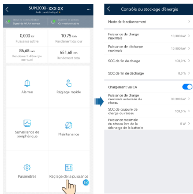
Figure 7-11 Réglage des paramètres de contrôle du stockage d'énergie
