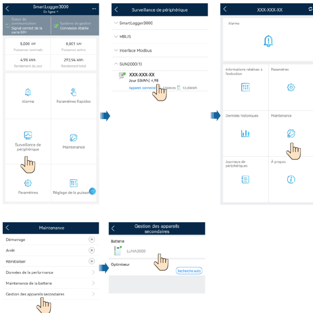
Figure 7-15 Recherche de l'état de la batterie
