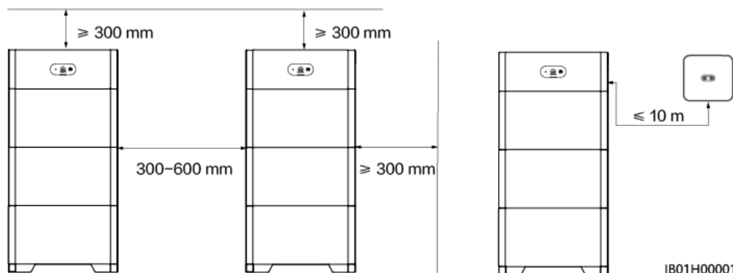
Figure 5-1 Espace d'installation
