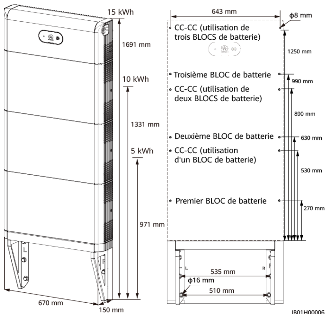
Figure 5-7 Dimensions d'installation murale
