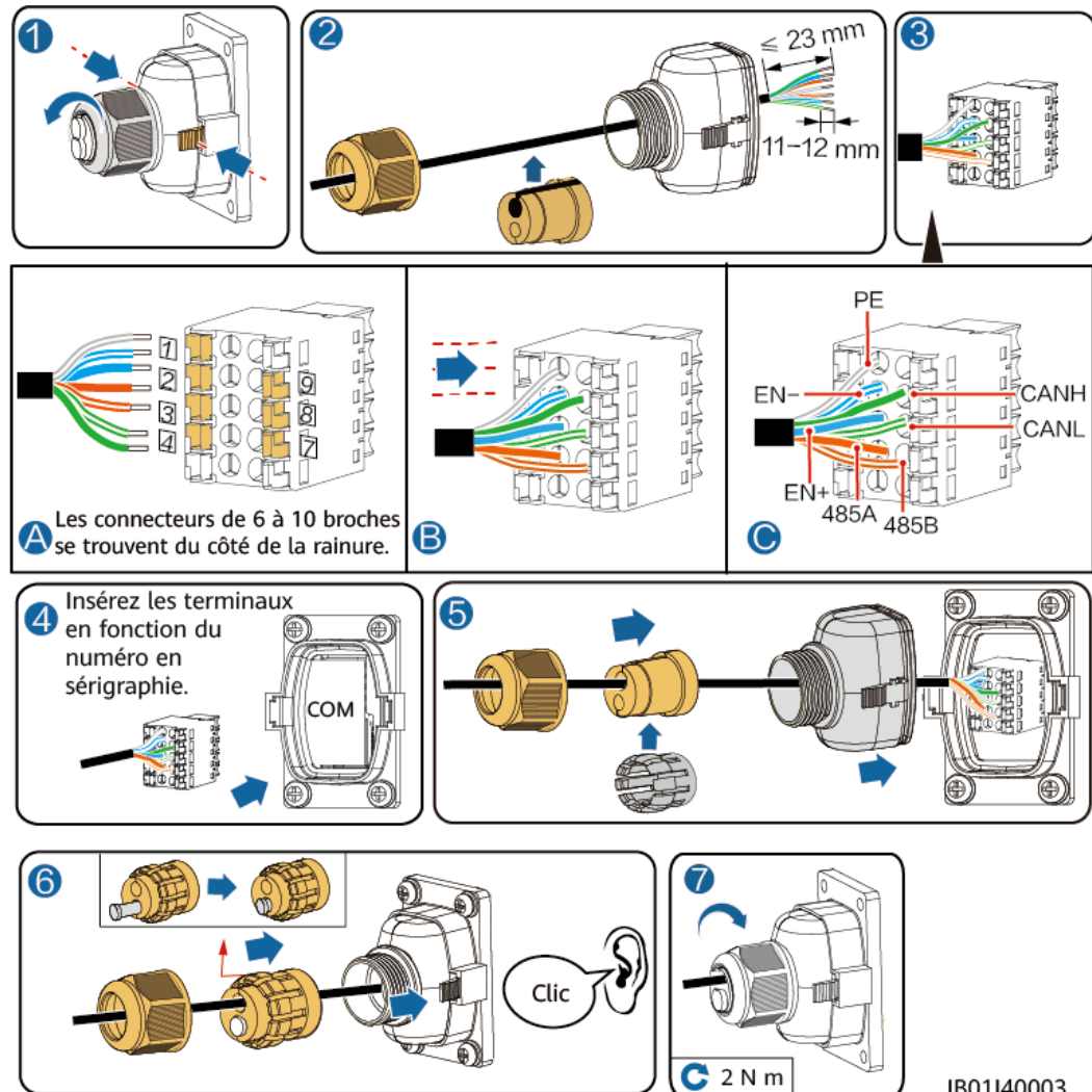
Figure 6-18 Installation d'une borne de communication en cascade
