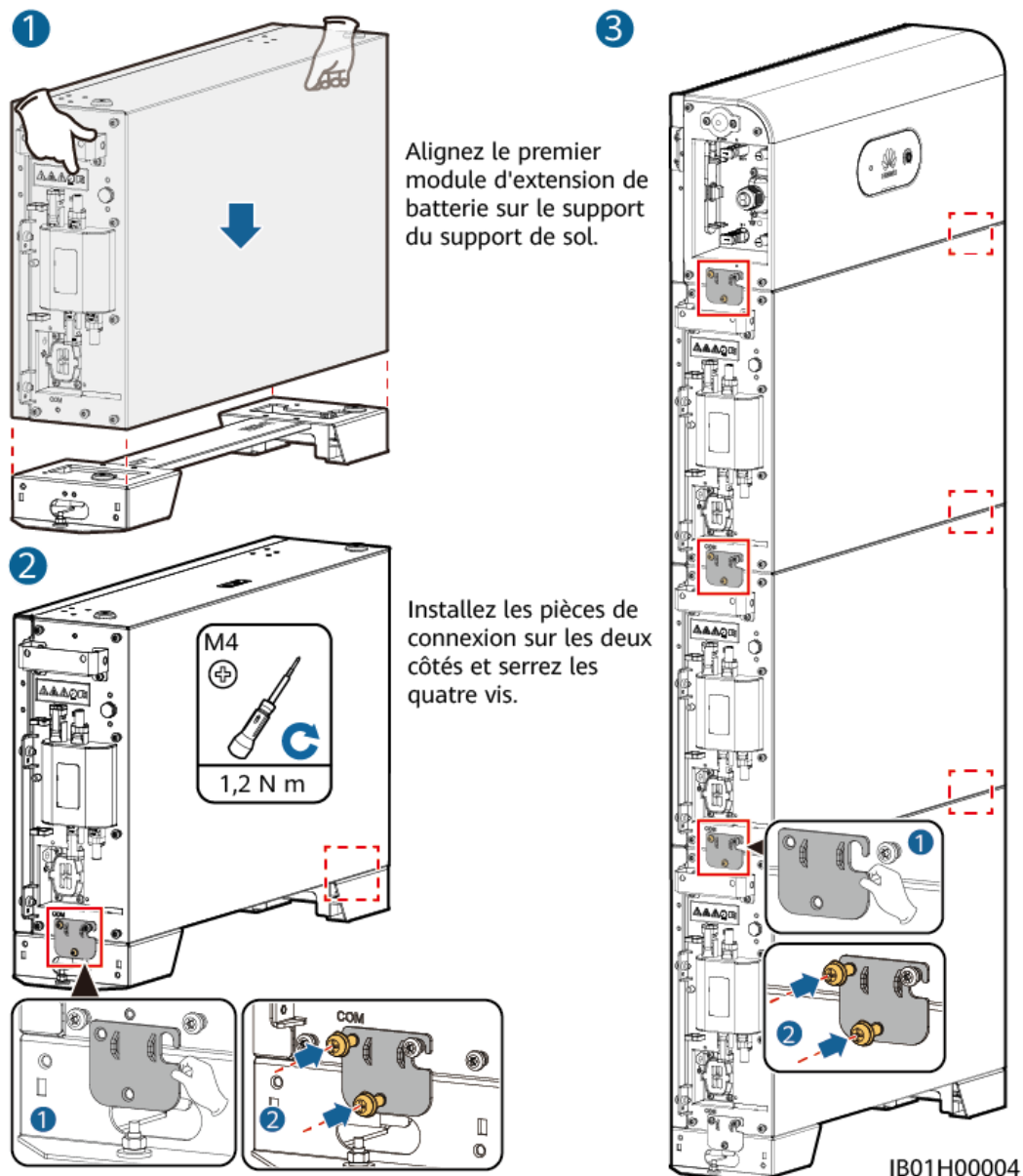
Figure 5-5 Installation des modules d'extension de batterie et du module de contrôle de l'alimentation
