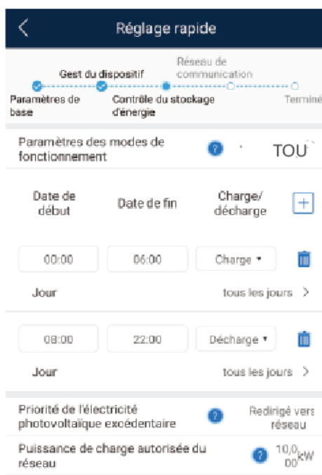
Figure 4-7 Mode de fonctionnement TOU (Prix selon le temps d'utilisation)
