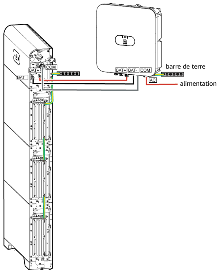
Figure 8-3 Schéma de raccordement des câbles
