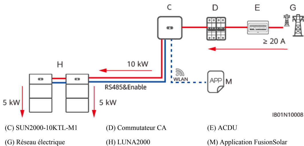
Figure 8-1 Schéma de mise en réseau pour un scénario de source d'alimentation triphasée
