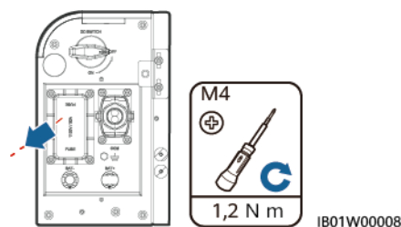
Figure 11-1 Retrait des vis de l'armoire
