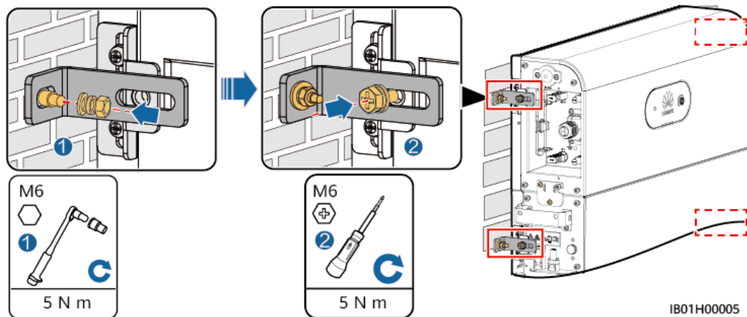
Figure 5-9 Fixation du module de contrôle de l'alimentation
