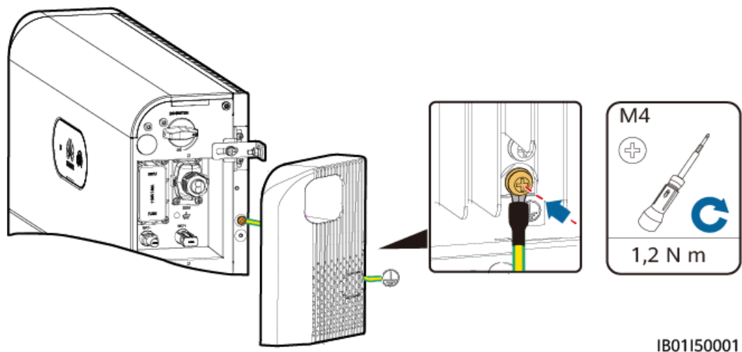
Figure 6-10 Mise à la terre du câble PE
