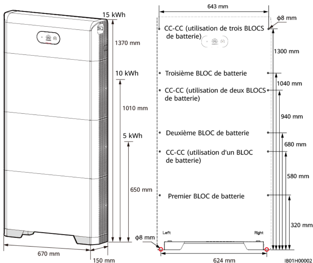
Figure 5-2 Dimensions d'installation au sol
