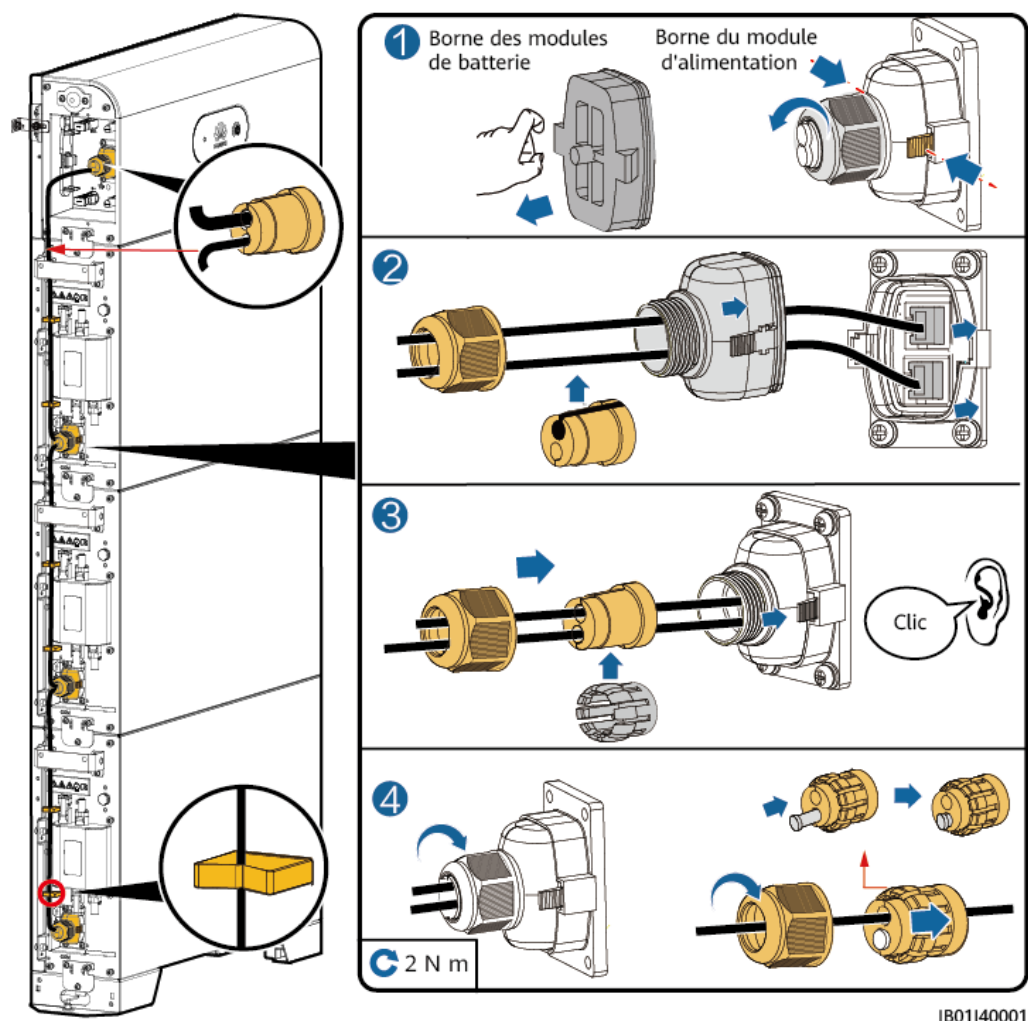
Figure 6-4 Fixation à l'aide d'attaches
