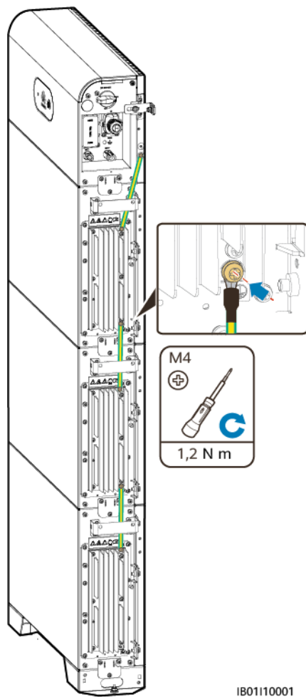
Figure 6-2 Raccordement du câble PE interne
