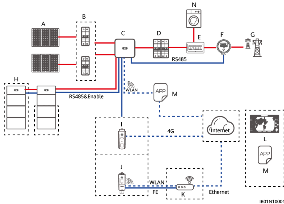
Figure 4-1 Schéma de mise en réseau ESS raccordé au réseau (composants optionnels indiqués par des encadrés en pointillé)
