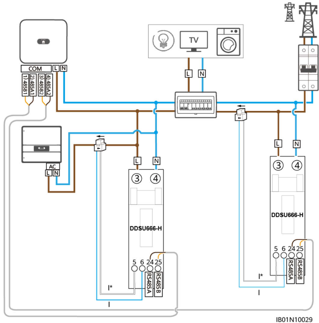
Figure 4-18 Raccordement des câbles du compteur électrique pour le SUN2000-(2KTL-6KTL)-L1
