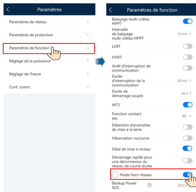
Figure 4-14 Paramètre de l'alimentation de secours
