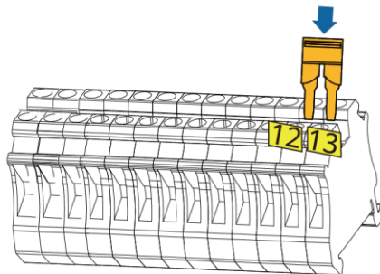
Terminale CA X3 dell'inverter (trifase)
