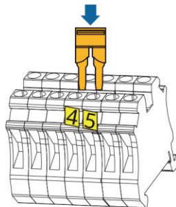
Terminale CA X2 per rete elettrica (monofase/trifase)
