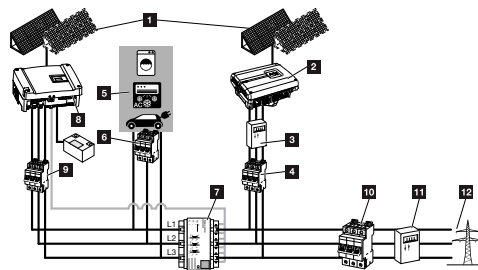
Afb. 4: Aansluiting van meerdere omvormers - stroomsensorpositie modus 2 voor netvoeding (mogelijk met PIKO BA van HW versie 040101)
