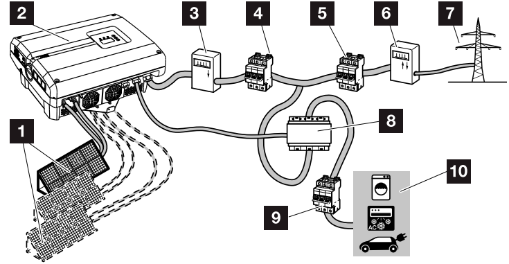
Abb. 8: Akım sensörlü fotovoltaik sistem
