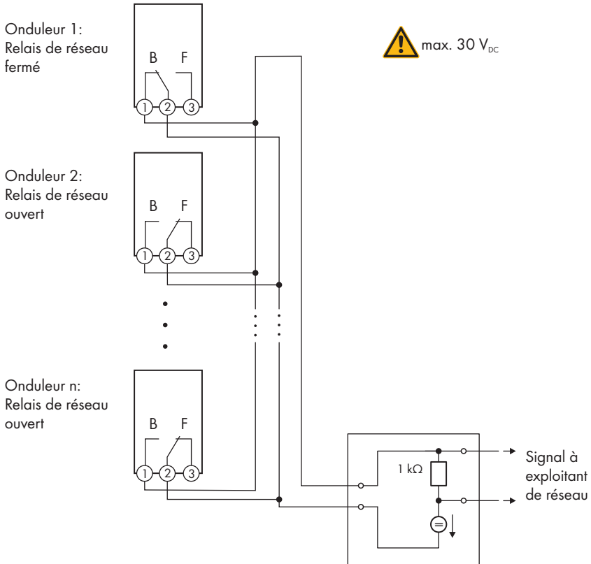
Figure 18 : Plan de raccordement pour le signalement de l'état de commutation du relais du réseau (exemple)
