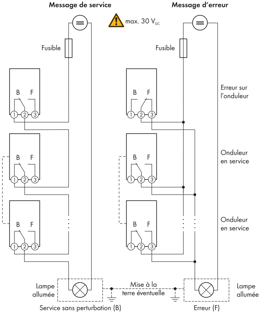
Figure 16 : Plan de raccordement avec plusieurs onduleurs en cas de raccordement d'un indicateur de fonctionnement et en cas de raccordement d'un indicateur d'anomalie (exemple)
