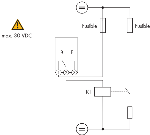
Figure 17 : Plan de raccordement pour la commande d'un appareil consommateur
