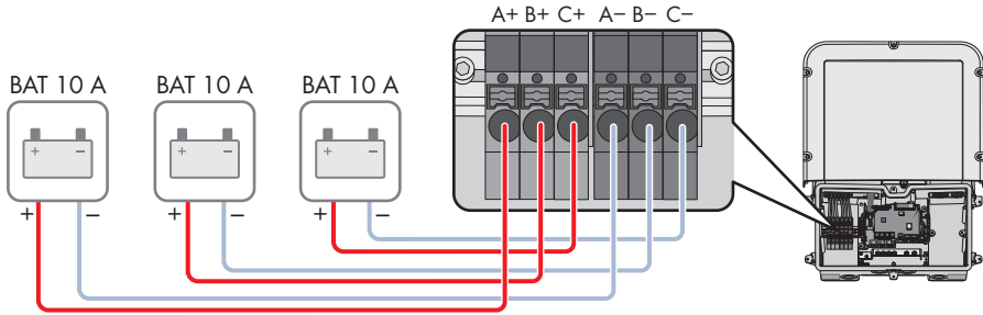
Figure 21 : Aperçu des connexions pour le raccordement de 3 batteries avec des courants de charge/décharge limités à 10 A chacune.
