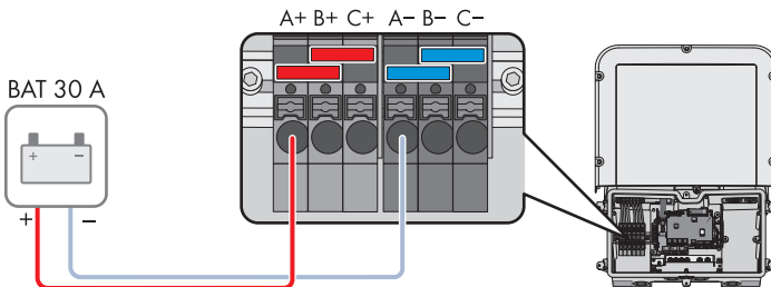
Figure 24 : Aperçu des connexions pour le raccordement d'une batterie dont le courant de charge/décharge est limité à 30 A
