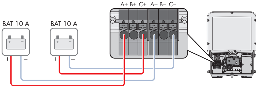
Figure 20 : Aperçu des connexions pour le raccordement de 2 batteries avec des courants de charge/décharge limités à 10 A chacune.
