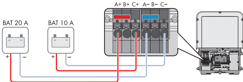
Figure 22 : Aperçu des connexions pour le raccordement de 2 batteries avec des courants de charge/décharge limités à des valeurs différentes.
