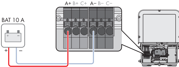
Figure 19 : Aperçu des connexions pour le raccordement d'une batterie dont le courant de charge/décharge est limité à 10 A
