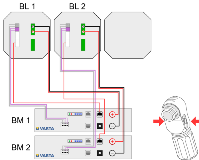
Abbildung 6: Batterielader 1 und 2, Batteriemodul 1 und 2
