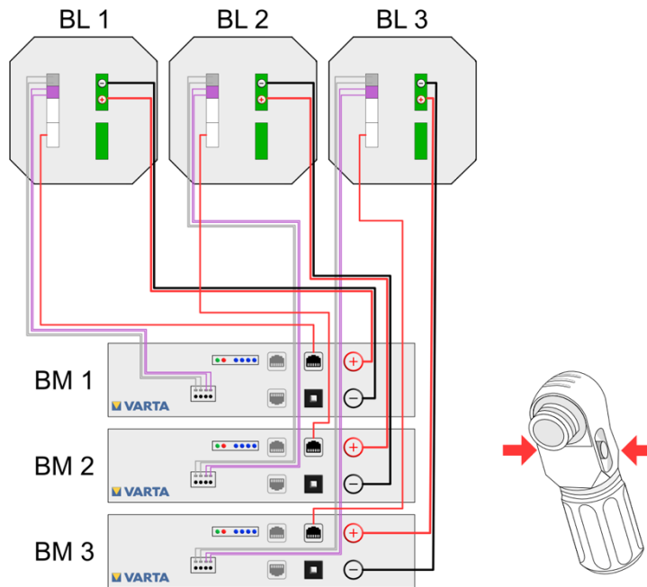
Abbildung 8: Batterielader 1 und 2, Batteriemodul 1, 2 und 3,
