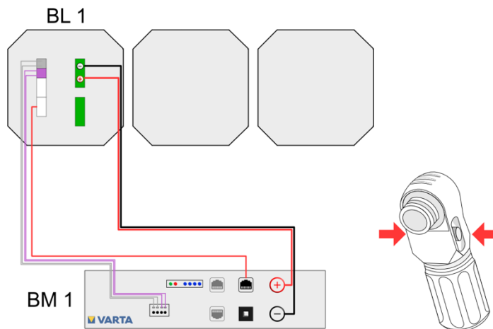
Abbildung 4: Batterielader 1 - Batteriemodul 1
