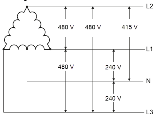
Fig. 4 Zweiphasensystem mit Nullleiter (3-drahtig)
