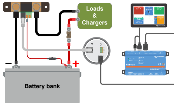
Il monitor della batteria è collegato a un Cerbo GX e a uno schermo GX Touch.
