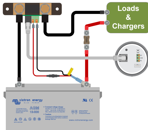
Monitor della batteria con rilevamento ausiliare della temperatura.
