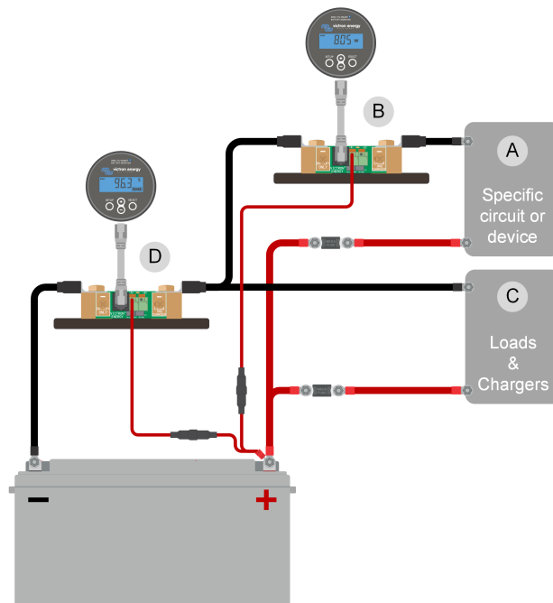
Esempio di sistema che comprende un monitor della batteria principale assieme a un monitor della batteria separato e configurato come monitor CC per monitorare un particolare dispositivo o circuito. Un monitor della batteria viene utilizzato come contatore di CC (B) e l'altro viene utilizzato come monitor della batteria (D).
