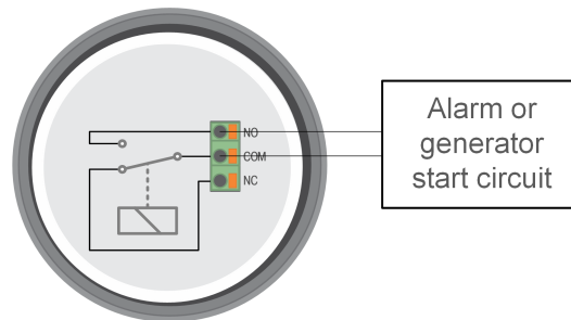
Schema di cablaggio interno del monitor della batteria con il relè in stato di diseccitazione collegato a un circuito esterno di allarme o di avvio del generatore.
