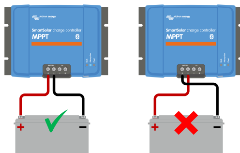
Esempi di polarità corretta ed erronea (inversa) della batteria.
