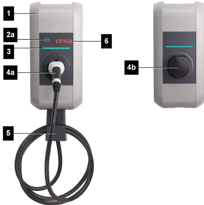
Abb. 3-1: Übersicht Ladestation
