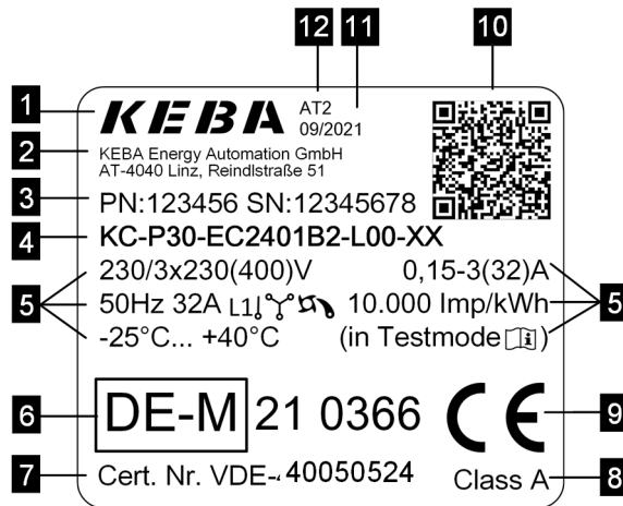
Abb. 4-7: Beispiel Typenschild
