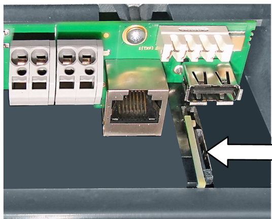
Fig. 8-22: Logement pour carte
